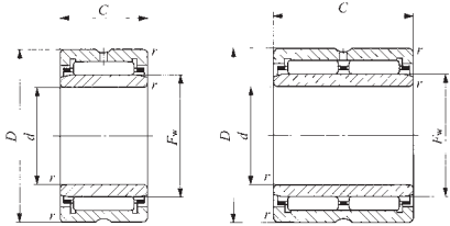
NA49 TAFI NA69( d \leq 30 ) NA69
